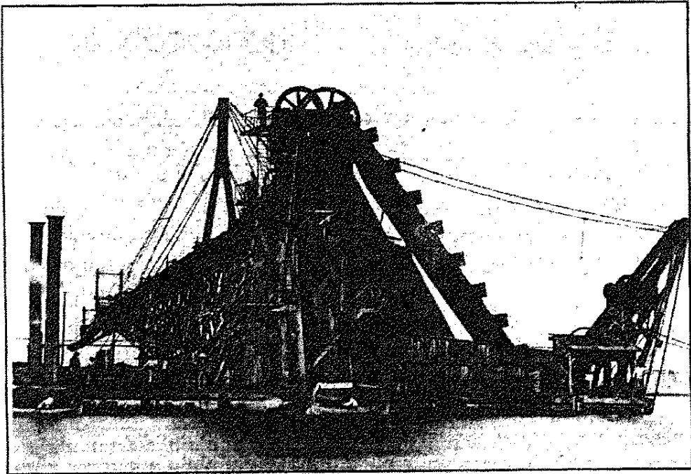
آخر جيل من الجرّافات بندراع طويل
